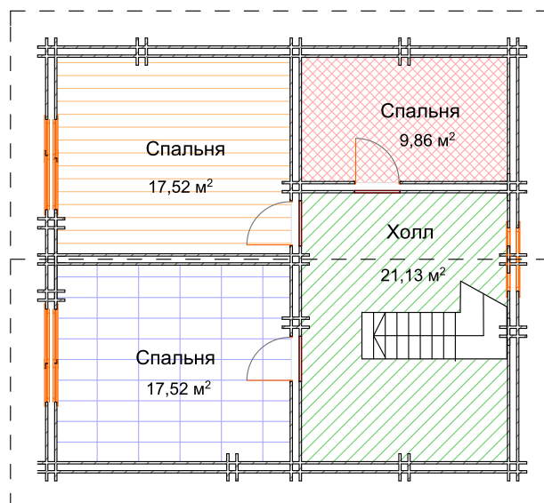
План помещений 2 этажа
