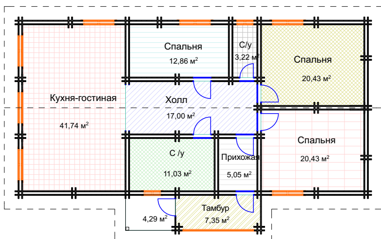
План этажа
