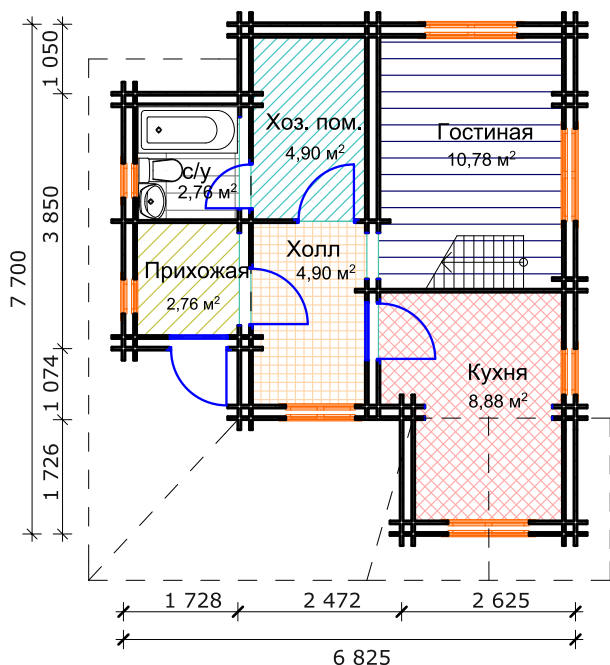
План помещений 1 этажа
