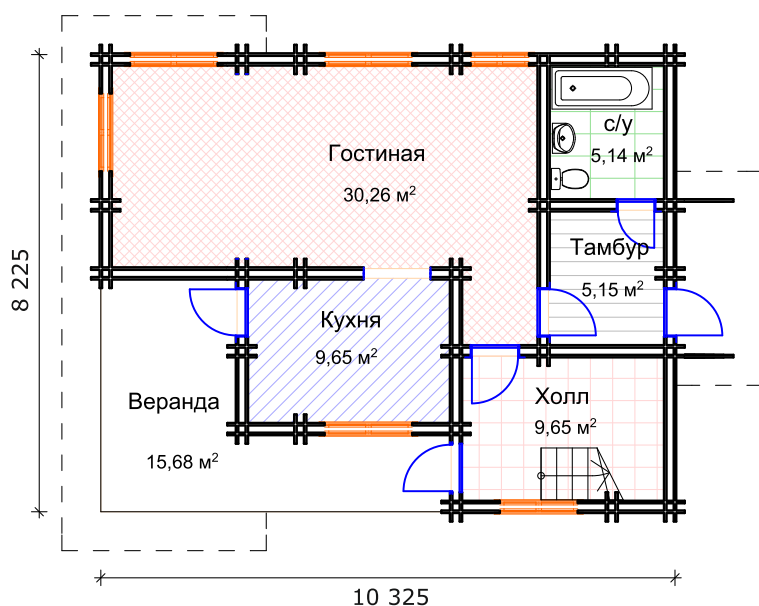
План помещений 1 этажа
