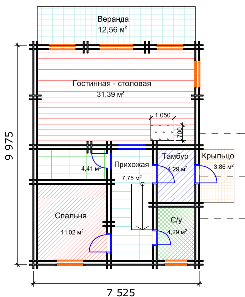
План помещений 1 этажа
