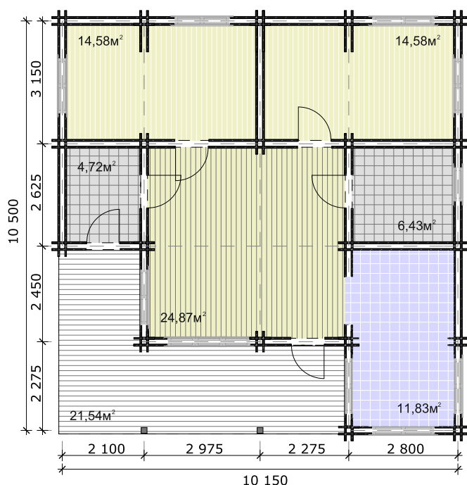
План помещений
