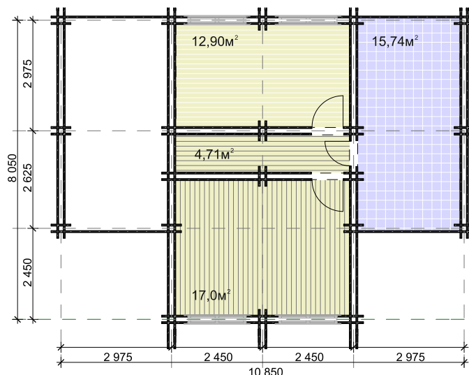
План помещений 2 этажа
