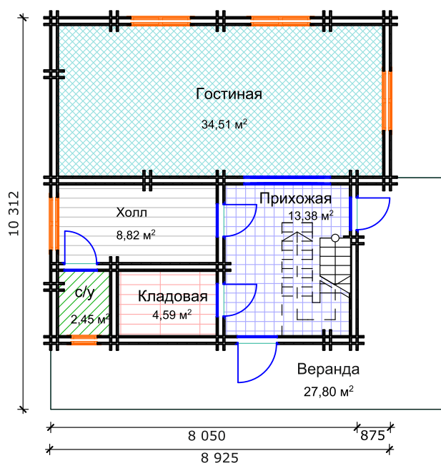
План помещений 1 этажа
