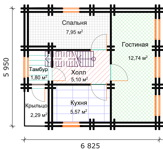
План помещений 1 этажа
