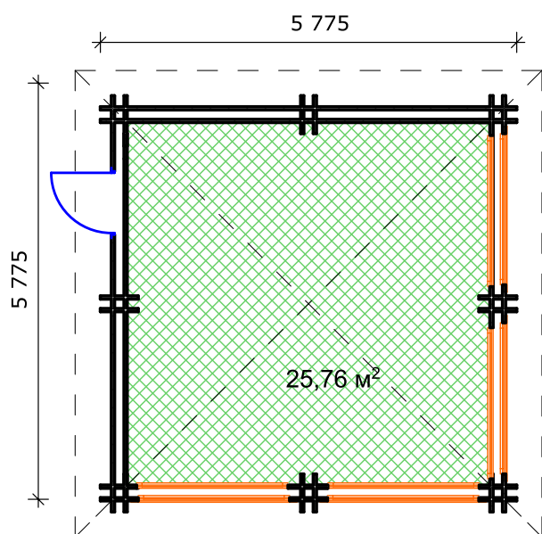
План помещения
