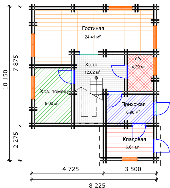
План помещений 1 этажа
