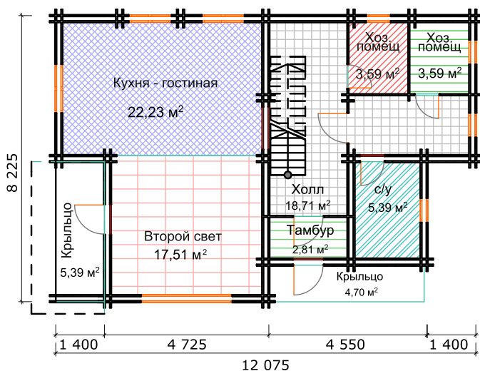
План помещений 1 этажа
